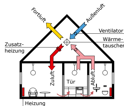
System einer kontrollierten Be- und Entlüftung.
