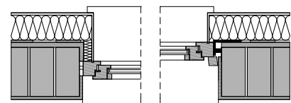
oben: Einbausituation Fenster
