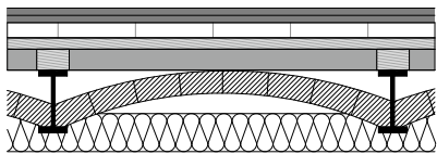
Sogenannte preußische Kappendecke aus Mauerwerk und Stahlträgern mit nachträglicher Dämmung von unten.
